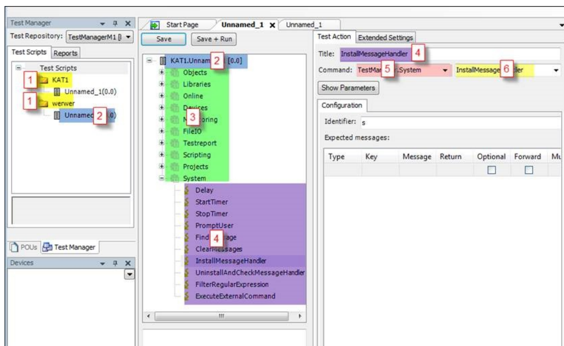
Bild 1: Terminologie: (1) Testkategorie, (2) Testsript, (3) Testfall, (4) Testaktion, (5) Befehlskategorie, (6) Befehl
